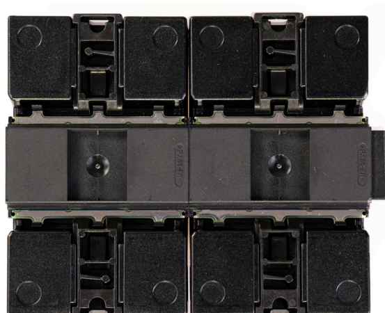
Fig.: Solar-Log Base e Solar-Log MOD 485 con connettore bus collegati.
