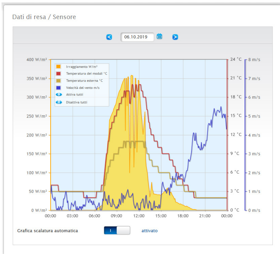
Fig.: Diagramma valori del Sensorbox
